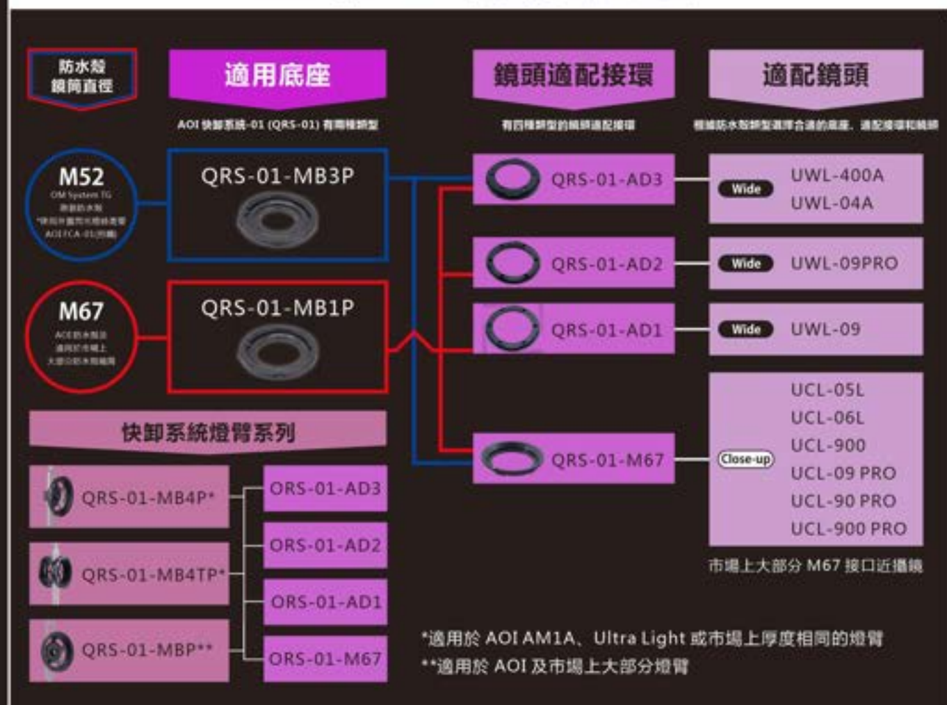
QRS-01-MB1P M67 防水殼快卸系統底座
